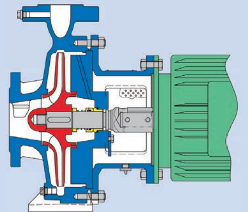
■ KRCB – в блочном конструктивном исполнении
