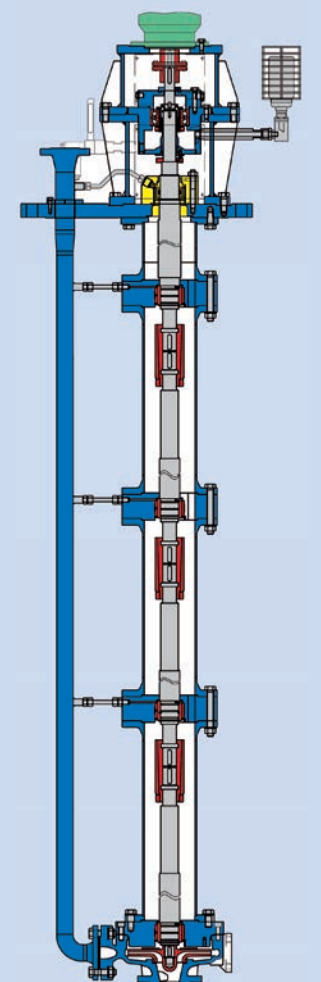
■ KRCV – в вертикальном конструктивном исполнении
