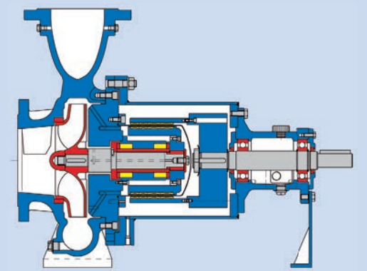
■ KRCM – с магнитной муфтой
